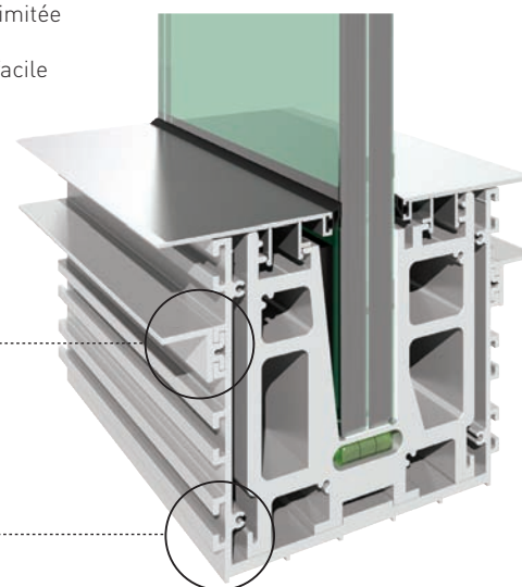
Height Adjusting U Case Profile Option Höhenstellprofil für U Gehäuse Option pour cadre réglable
